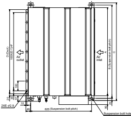
SEZ-Kanaleinbaugeräte, Kühlen/Heizen, SEZ-KD25-71VA
