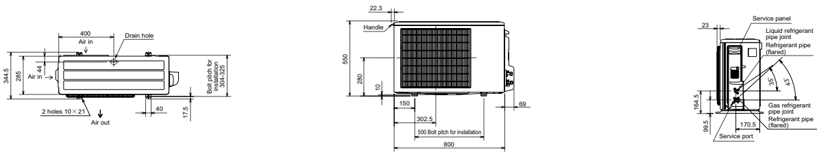
MUZ-Inverter Außengeräte, Kühlen/Heizen, MUZ-SF25-42VE
