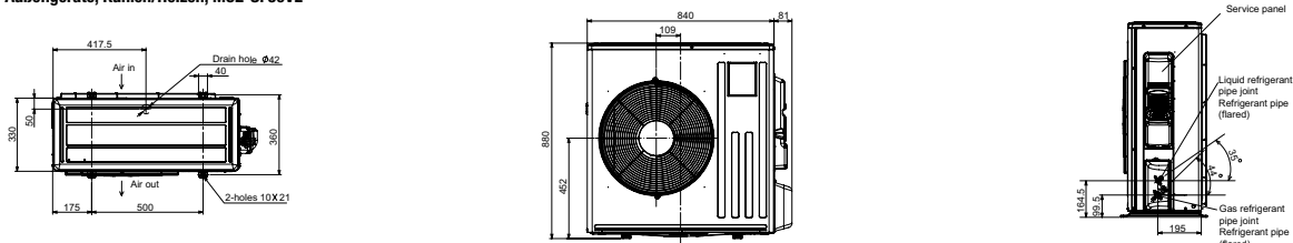
MUZ-Inverter Außengeräte, Kühlen/Heizen, MUZ-SF50VE
