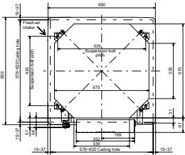
SLZ-4-Wege-Deckenkassetten, Kühlen/Heizen, SLZ-KA25-50VA
