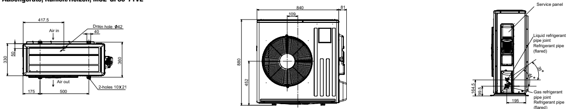
MUZ-Inverter Außengeräte, Kühlen/Heizen, MUZ-GF60-71VE
