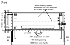
MLZ-1-Wege-Deckenkassetten, Kühlen/Heizen, MLZ-KA25-50VA
